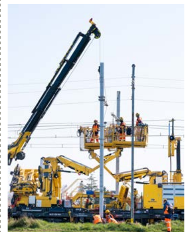
TSO-Zug erneuert Oberleitungen im 1.500-Volt-Netz
